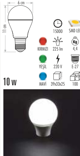
CT-4059 ALEV AMPUL (3 FONKSİYONLU)
