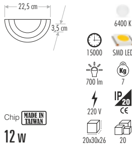
CT-5156 YARIM AY LEDLİ APLİK SIVA ÜSTÜ
