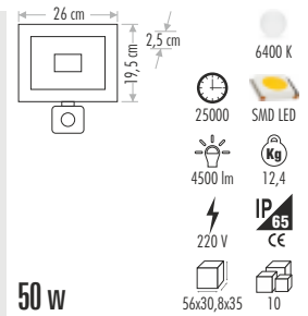
CT-4654 SENSÖRLÜ SLİM LED PROJEKTÖR 230,00 ₺
