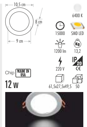
CT-5352 5" CLASS LED ARMATÜR YÜKSEK TAVAN 300,00 ₺
