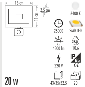
CT-4652 SENSÖRLÜ SLİM LED PROJEKTÖR 145,00 ₺
