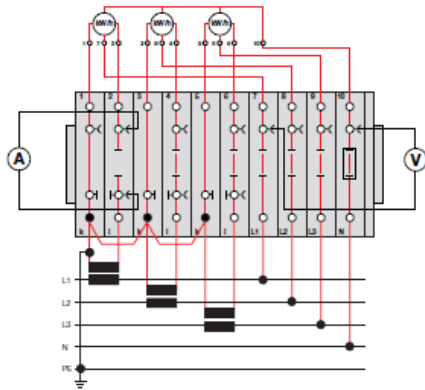
L1 için Örnek Ayırma ve Ölçme Şeması
