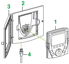
ATV71 uzaktan bağlantı kiti
