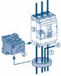
① Toroid ② Vigirex röle ③ MX bobini ④ Nötr
